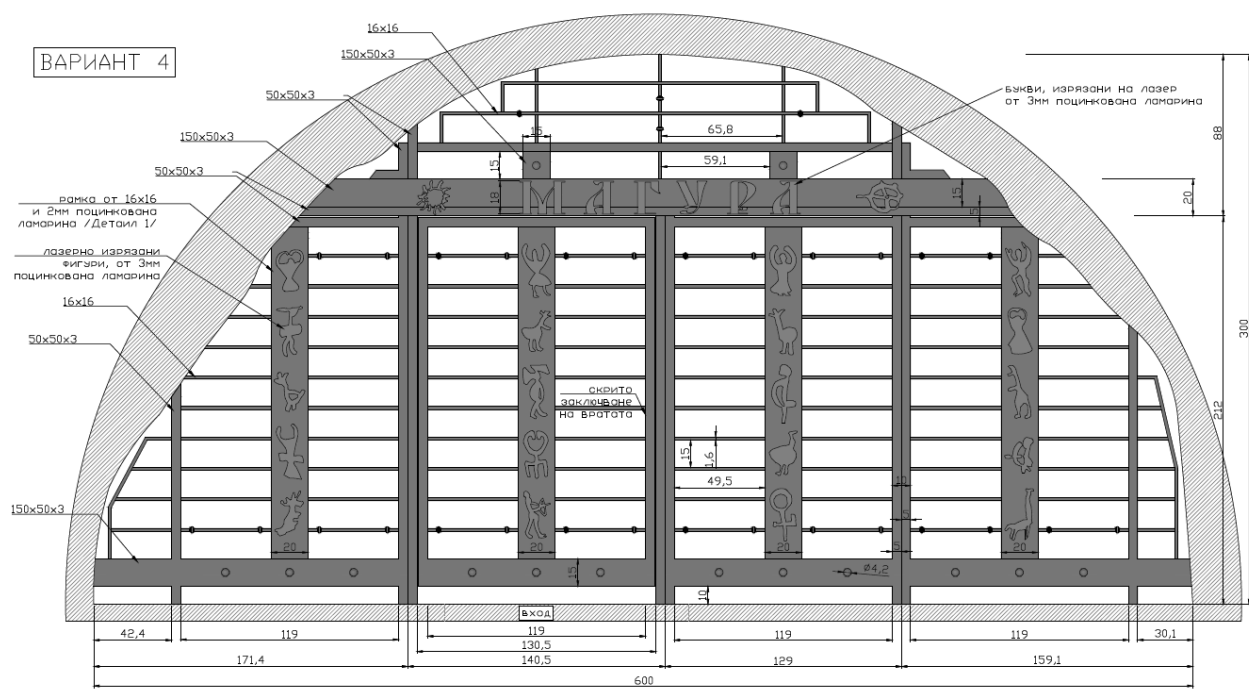
Схема с размери – входна врата
